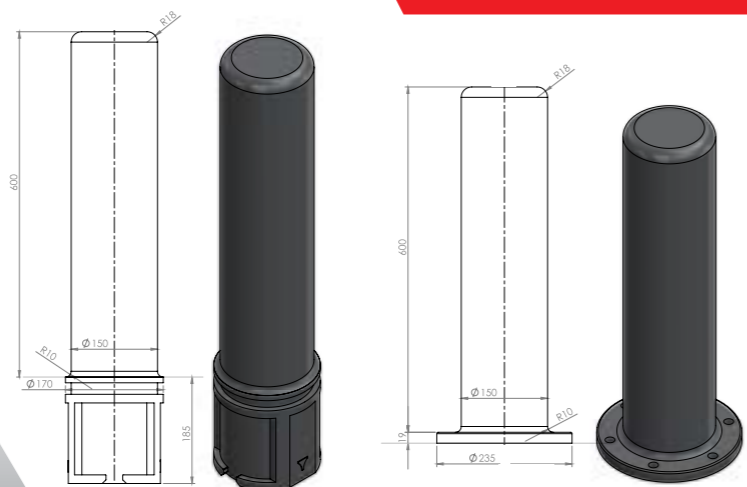
מק"ט 600001 התקנה עם ברגים מק"ט 600005 התקנה ביציקת בטון
